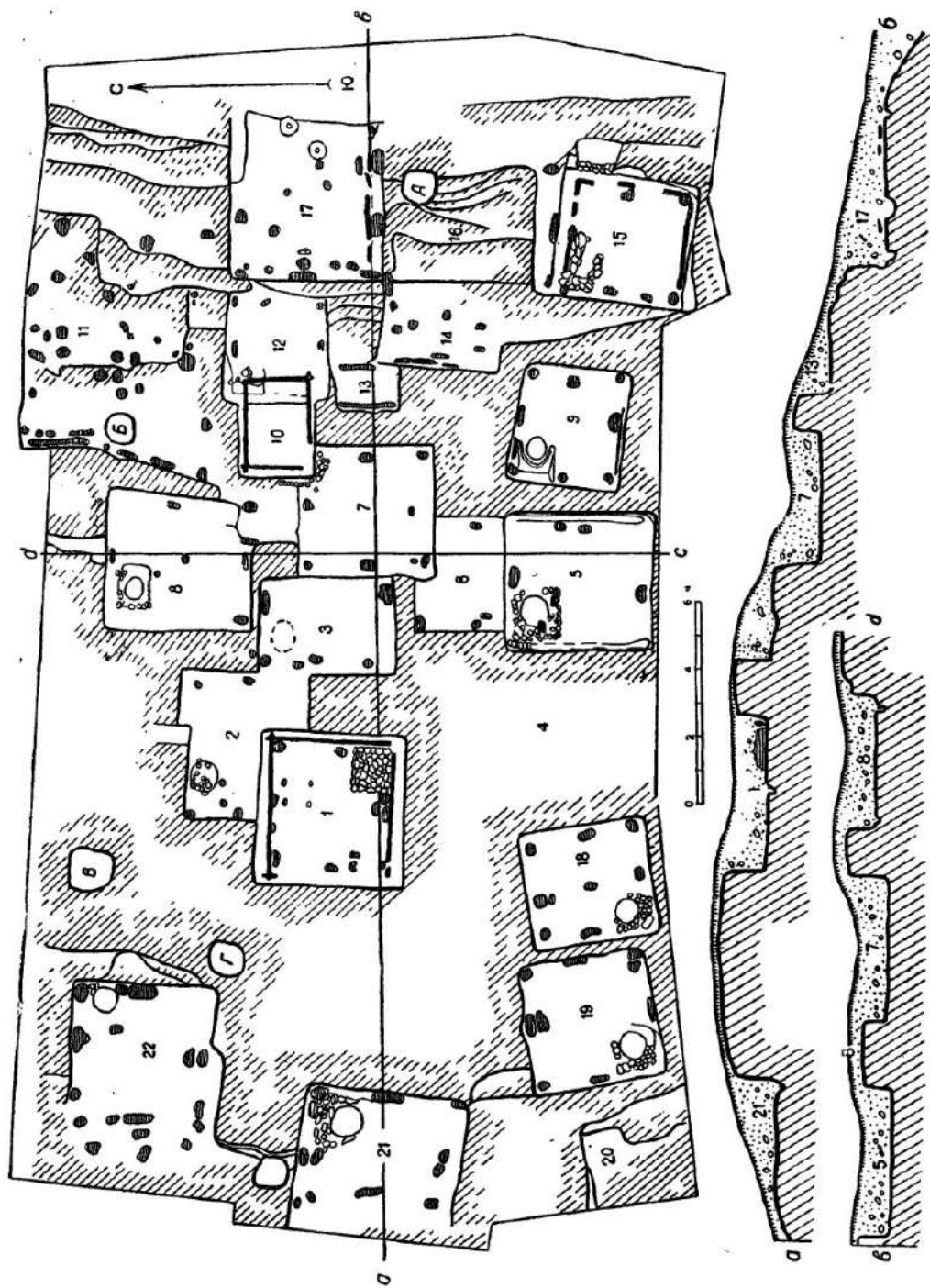
Рис. 115. План и разрезы расположеня жилищ Боршевского городища (раскопки П. П. Ефременко).
