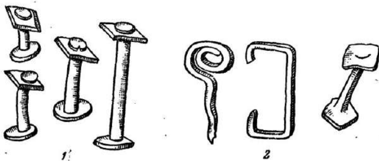
Рис. 187. Ладейные заклепки, скобы и пробой: 1 — Гнездово, 2 — Приладожье.
