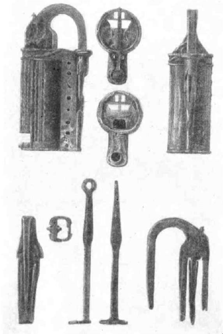
Рис. 143. Замки и ключи XII—XIII вв., найденные в Московском Кремле (по Солнцеву).
