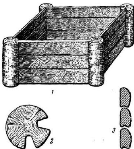
Рис. 102. Кожшевенный чан: 1 — общий вид; 2—3 — детали (Новгород. Раскопки А. В. Ардиховского).
