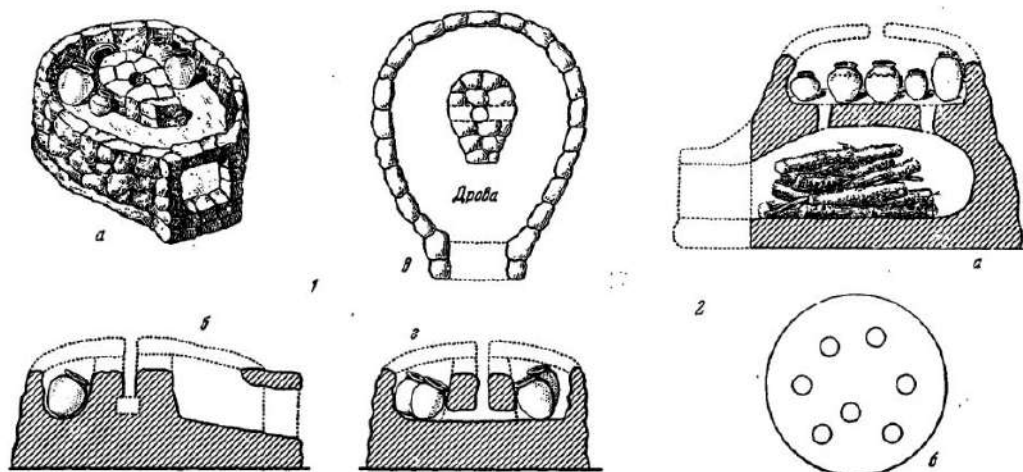
Рис. 96. Гончарные горны: 1 — горн, открытый раскопками в Белгороде: а — общий вид; б — продольный разрез; в — вид сверху; 2 — горн Донецкого городища: а — разрез; б — вид сверху на под горна.
