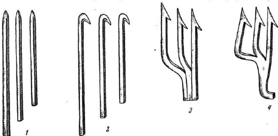
Рис. 48. Стадии изготовления остроги (изготовление вещи путем простейшей сварки): 1 — выковка стержней; 2 — загиб конца; 3 — заострение конца и сварка; 4 — готовая острога.
