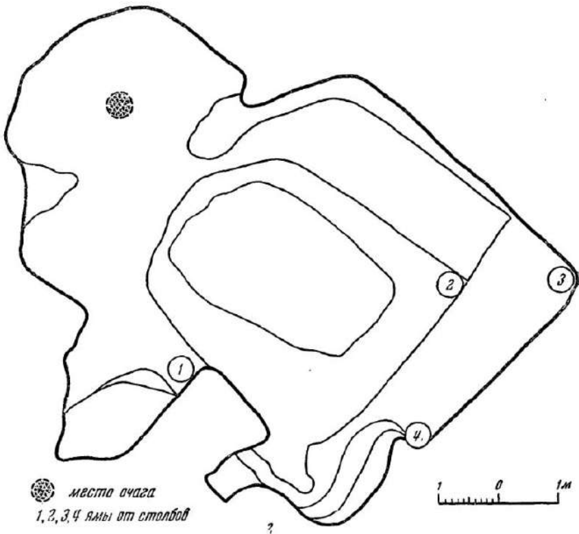
Рис. 128. Полуземляночное жилище (Суздаль. Раскопки А. Ф. Дубышина); 1— реконструкция, 2 — план.
