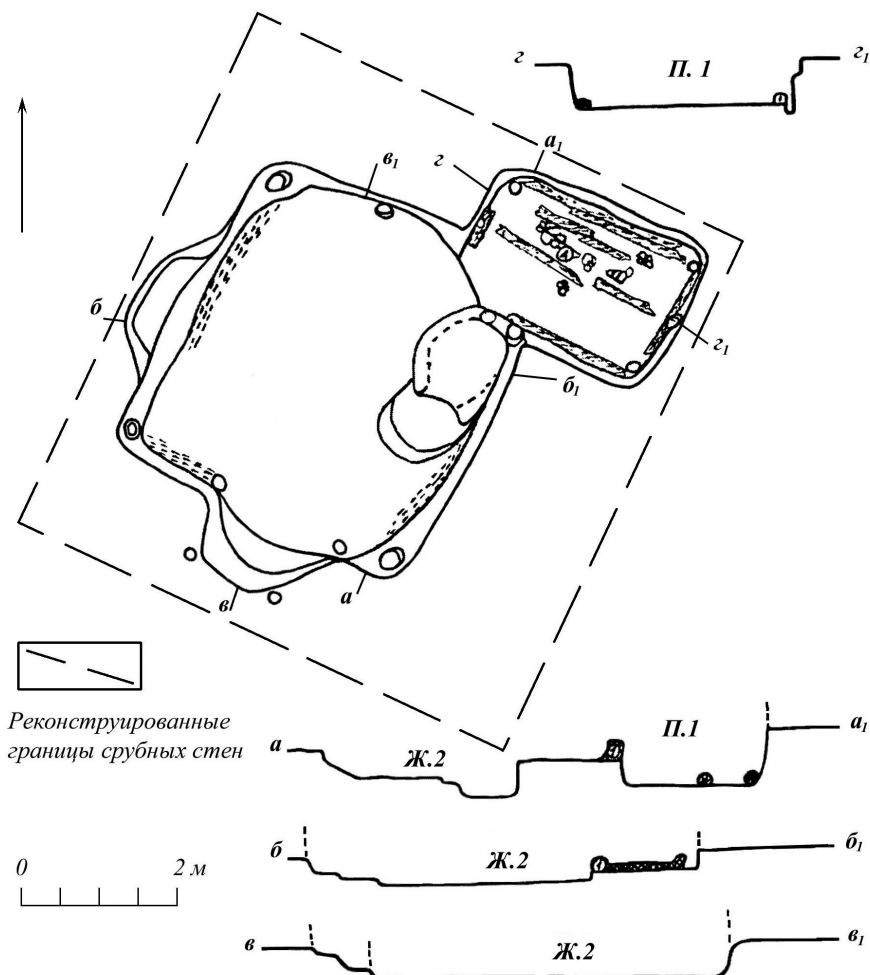
Рис. 1. Каменное, селище, жилище 2 и постройка 1 (по О.В. Сухобокову, с дополнениями)
